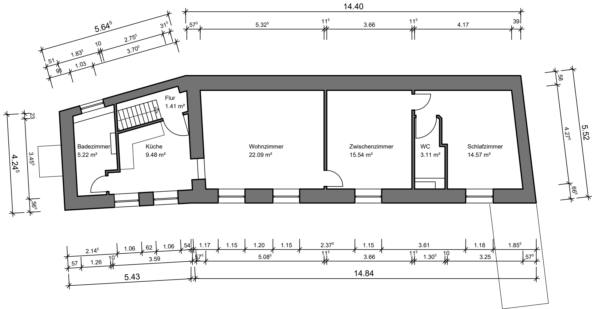
Obergeschoss M 1:100 Katzhecke 19, 52222 Stolberg
